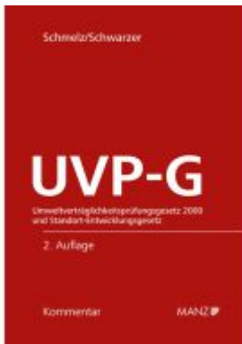
UVP-Gesetz Umweltverträglichkeitsprüfungsgesetz 2000
