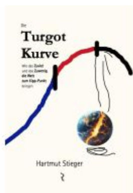
Die Turgot-Kurve
