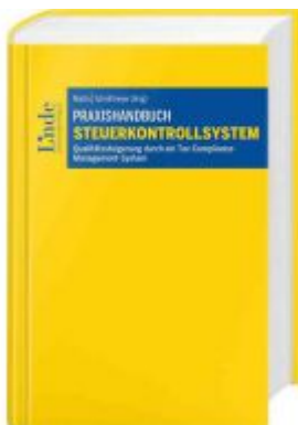
Praxishandbuch Steuerkontrollsystem
